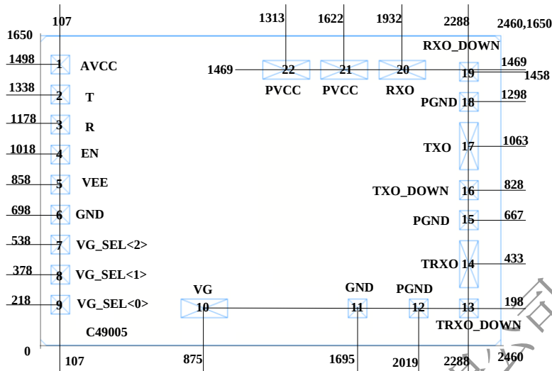
图 2 引脚分布图
