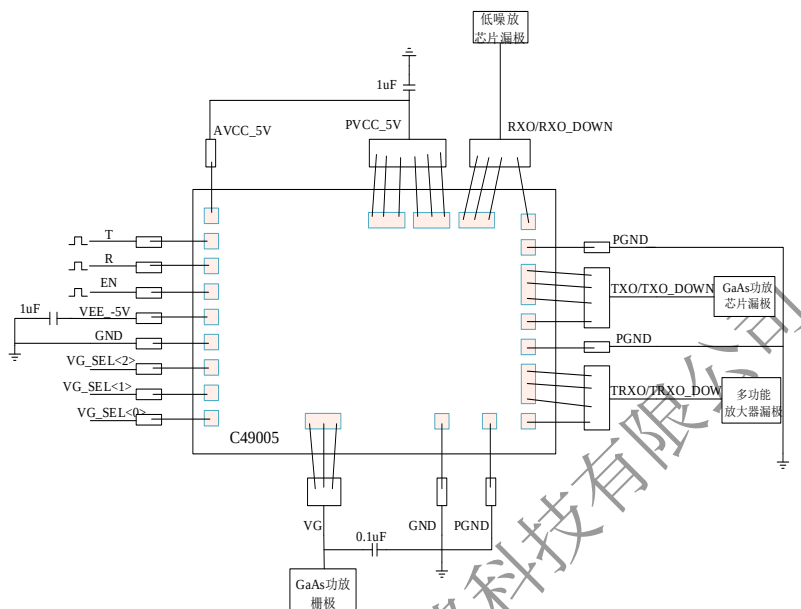
图 3 C49005 工作推荐电路
