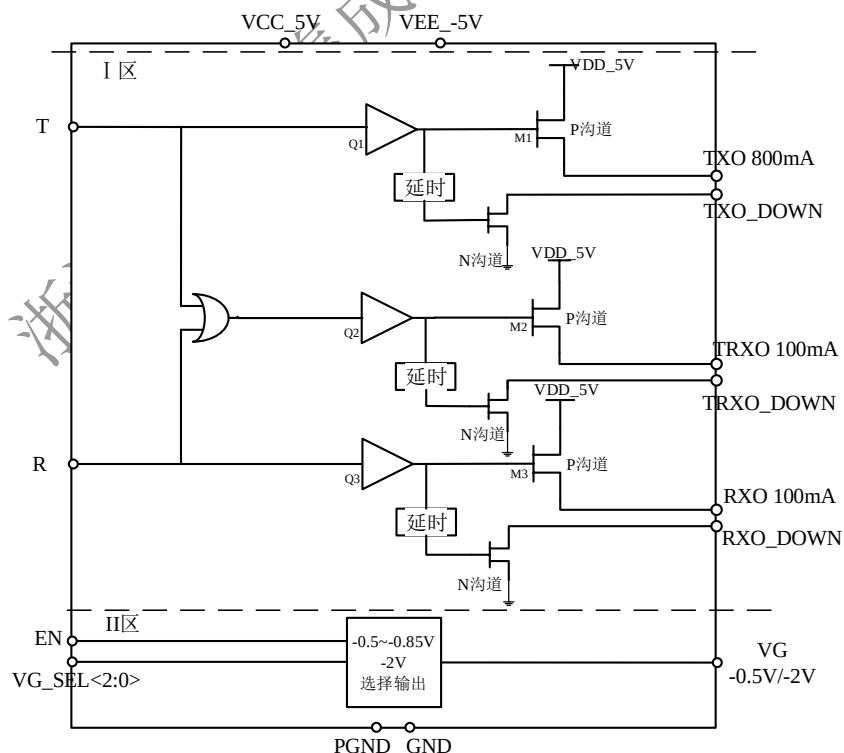
图 1 功能框图
