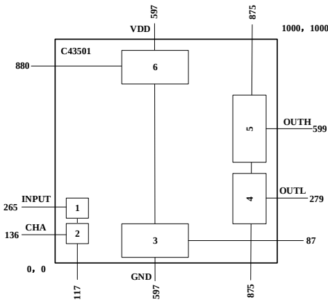
图 3 引脚分布图
