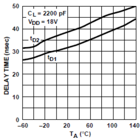
图 5 延迟时间
